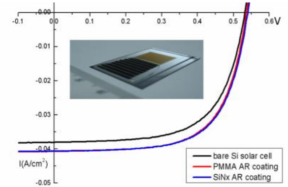
圖一 具奈米壓印抗反射結構與具一般單層SiN鍍膜之太陽能電池之電壓-電流特性比較
