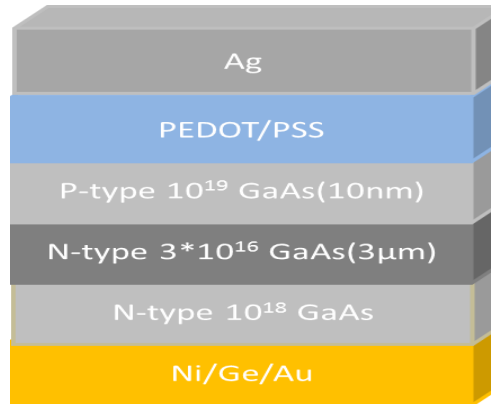
圖三 利用覆晶技術製作薄膜 PEDOT:PSS/GaAs 異質接面太陽能電池。
