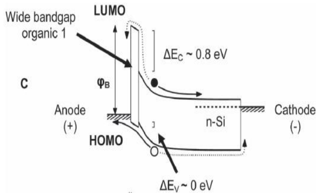
圖二 EDOT:PSS/Si 異質接面太陽能電池。
