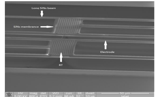
圖四 以奈米微影技術製作熱導測量元件，並進行單根有機(P3HT)及無機( Sb_2Se_3 )奈米線及奈米線束的熱導係數量測
